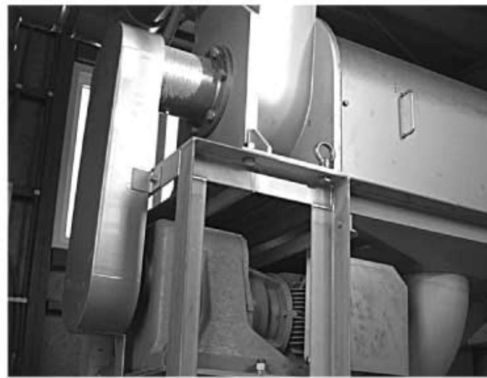
(上)家畜の尿と糞を区別する固液分離機 (左)メタンガスを一次的にバックに貯留 (左下)ガス発生を促進する大型ボイラー (下)発電のかなめ、駆動エンジン (最下)スラリーストアー
